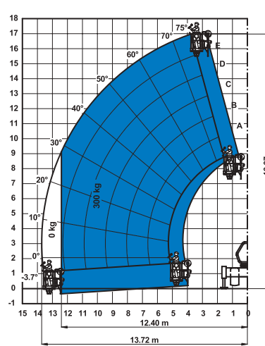
Su stabilizzatori con navicella fissa
