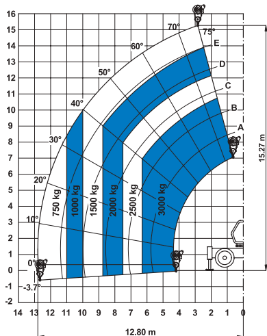
Su stabilizzatori con verricello idraulico 3 T
