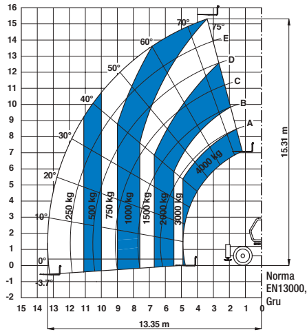
Su ruote con forche
