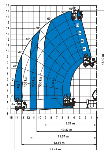
Su stabilizzatori con navicella girevole ed estensibile
