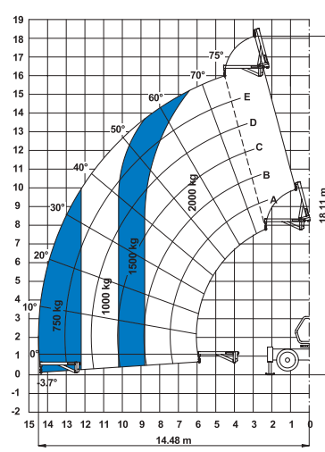
Su ruote con falcone 2 m (meccanico)
