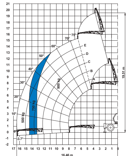
Su stabilizzatori con falcone 4 m (meccanico/idraulico)
